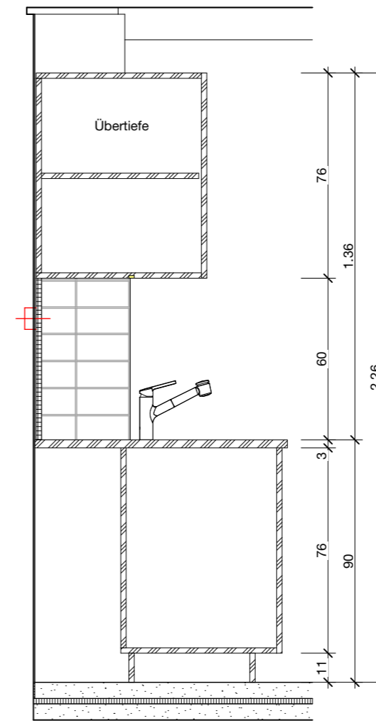
Schnitt A-A
