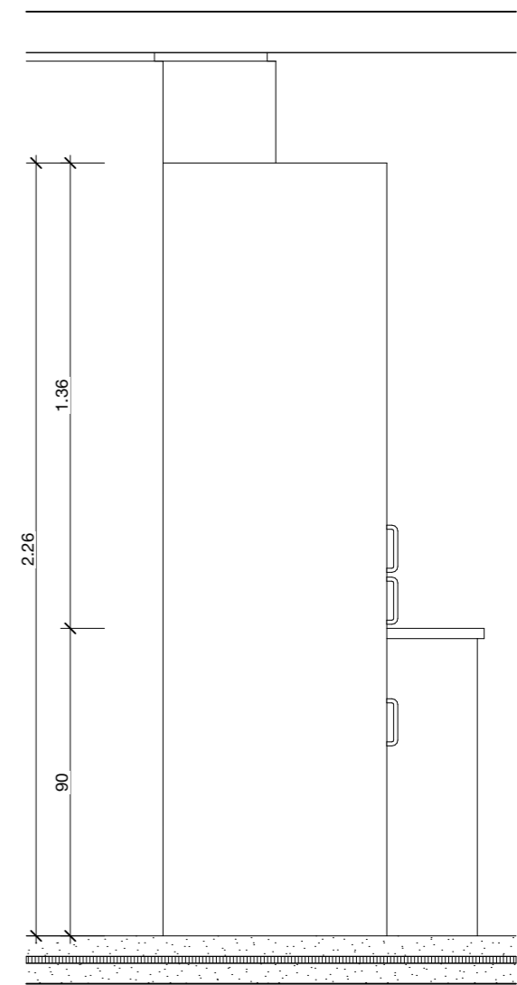
Ansicht B
