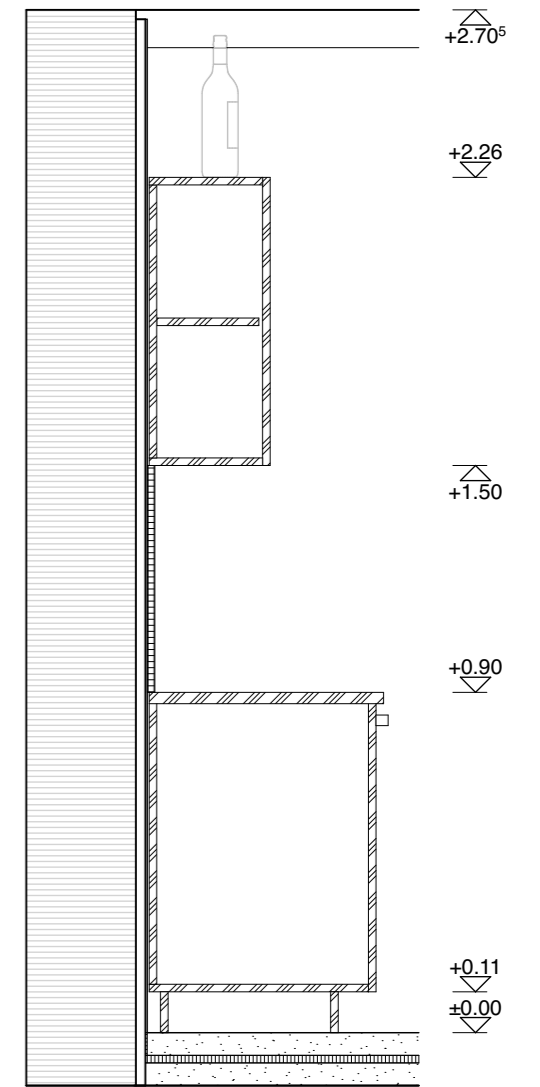
Schnitt B-B
