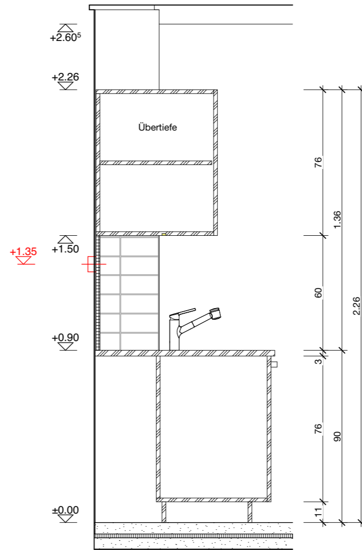
Schnitt A-A
